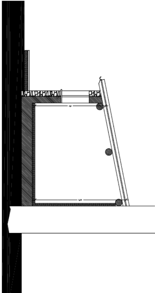
Sezione A-A'
